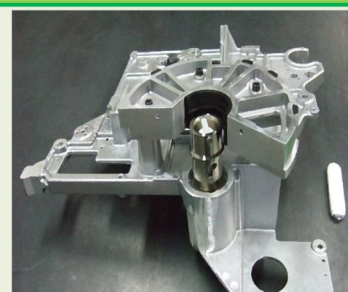
材質:ADC12 精度:位置度10μm
